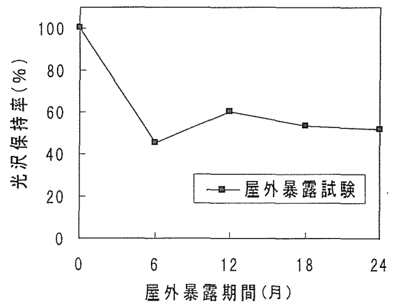
図17 造膜型における屋外暴露試験による光沢度変化
