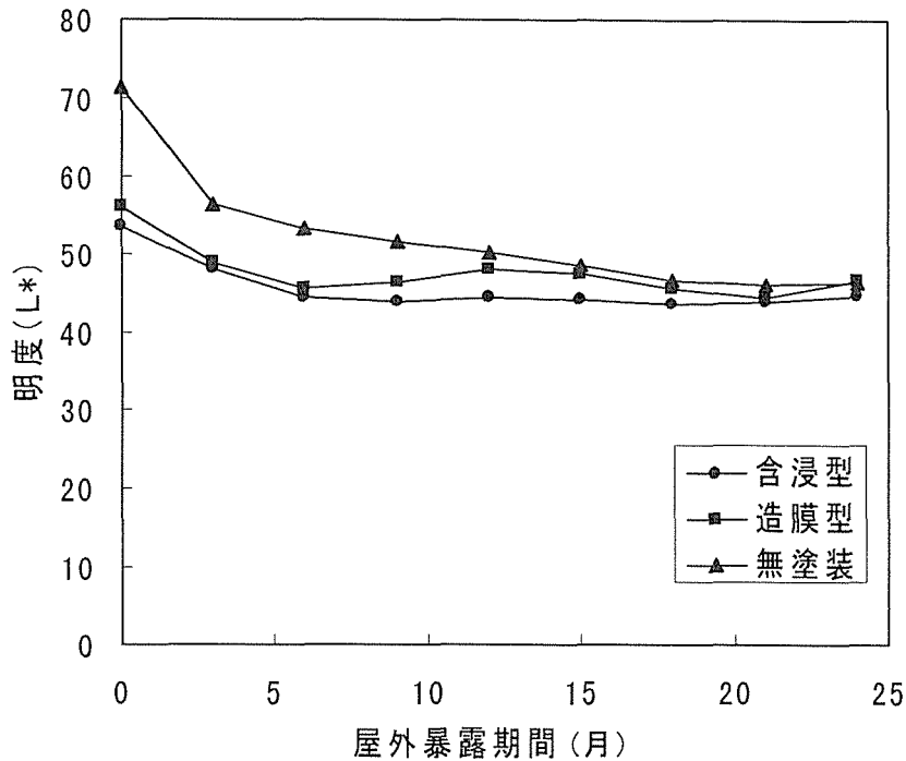
図8 屋外暴露試験による塗料タイプ別の明度変化
