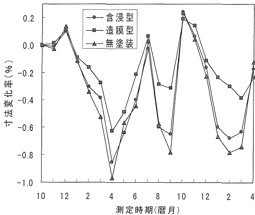
図20 屋外暴露における塗装木材の半径方向寸法の季節的变化
