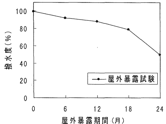
図19 含浸型における屋外暴露試験による撥水度変化
