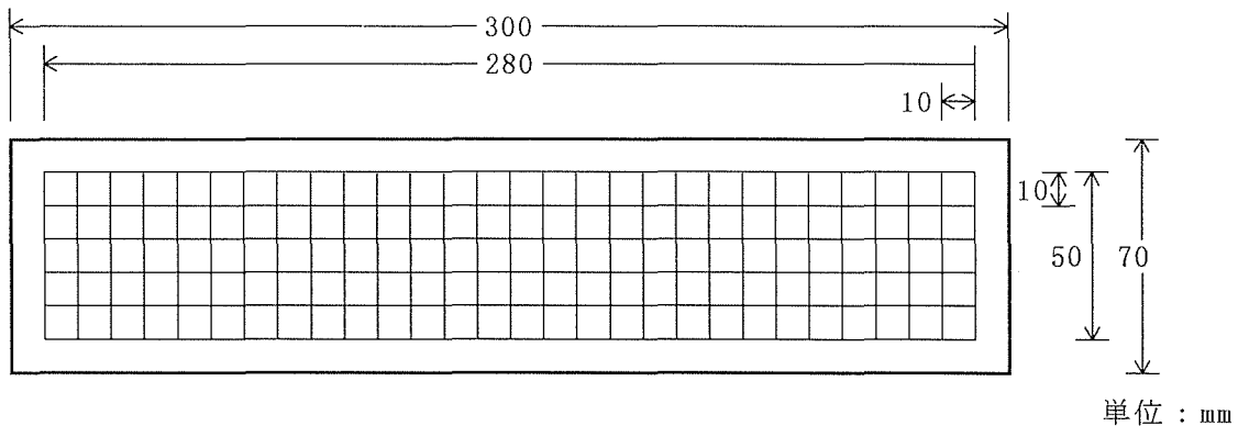
図1 塗膜欠陥率測定用シート（屋外暴露試験評価用） 注）試験片の周囲から10mm以内の部分は観察対象としない。
