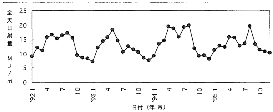
図6 暴露試験地付近の月間全日射量(1992/1-1995/12)
