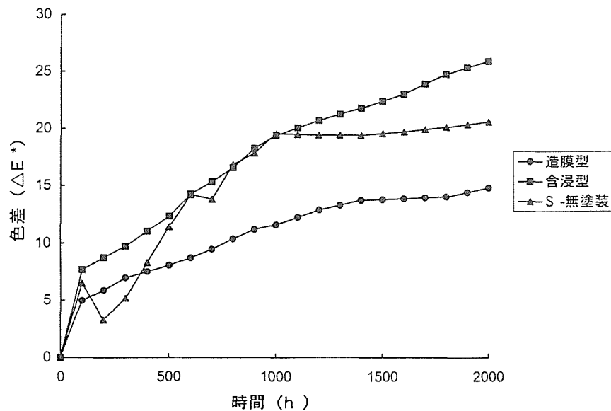
図4 促進耐候性試験による色差変化例
