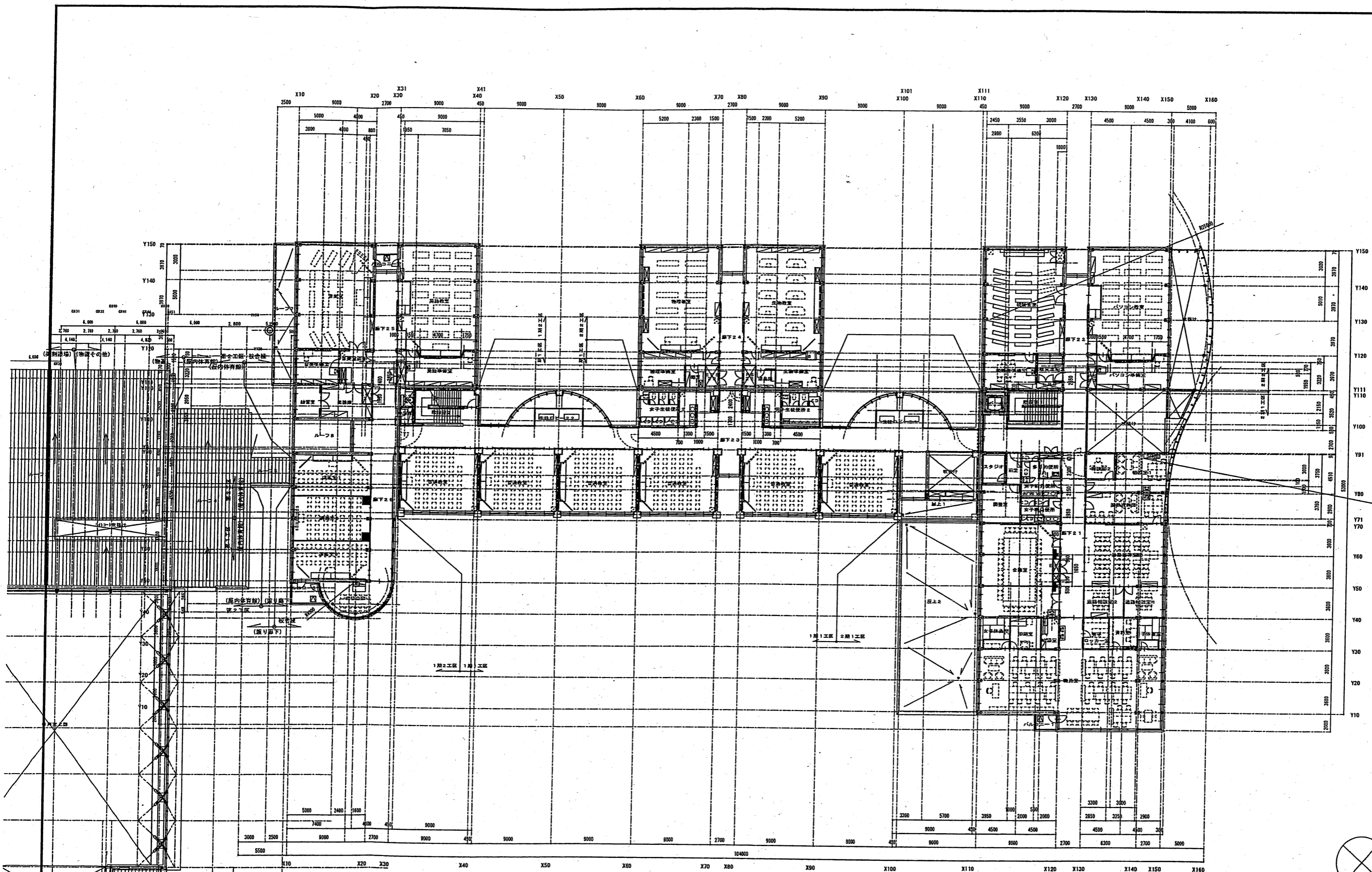
2階平面図 縮尺 1:200
