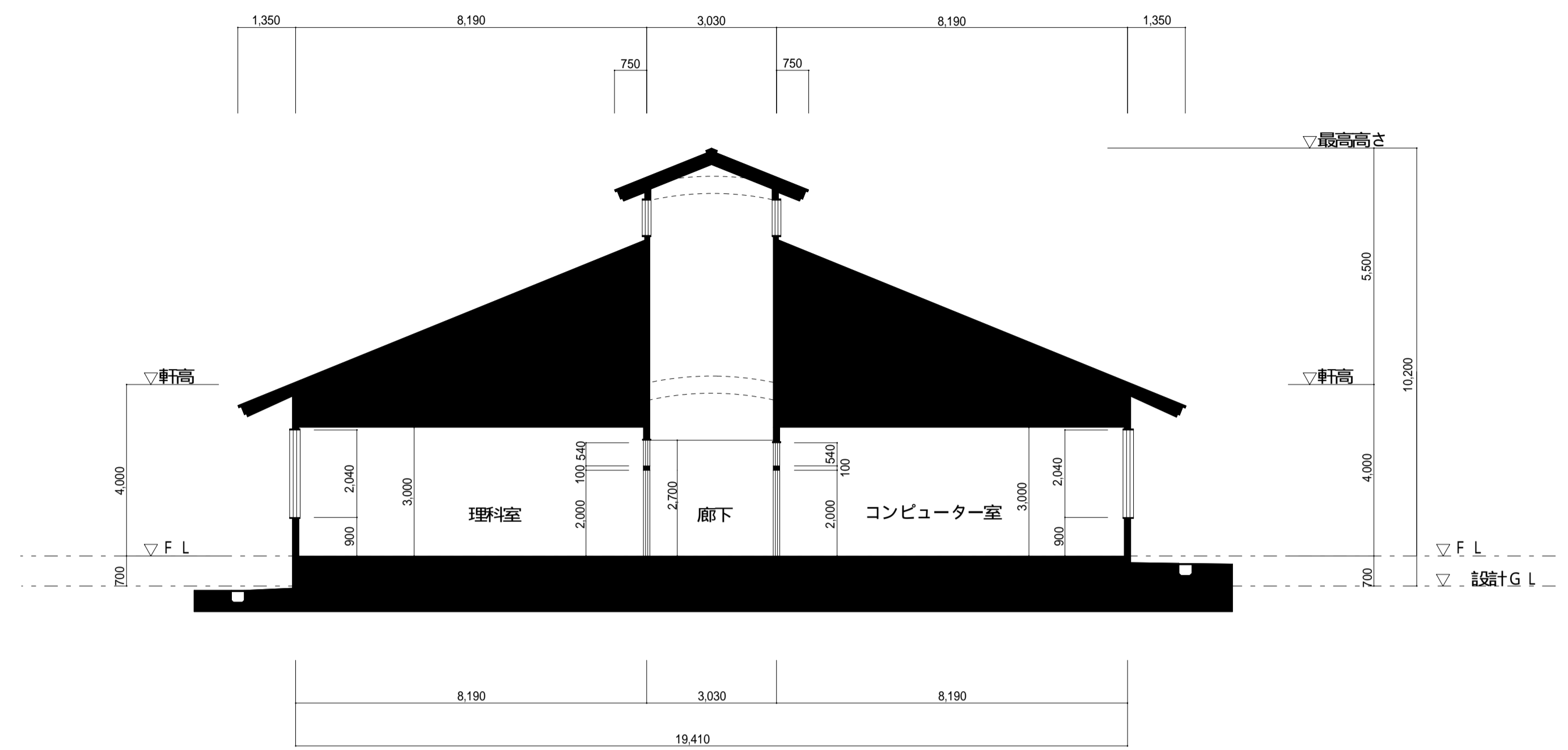
特別教室棟 B-B断面図
