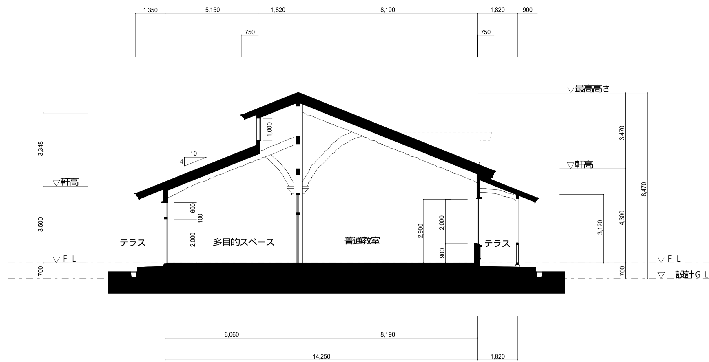
普通教室棟 A-A断面図
