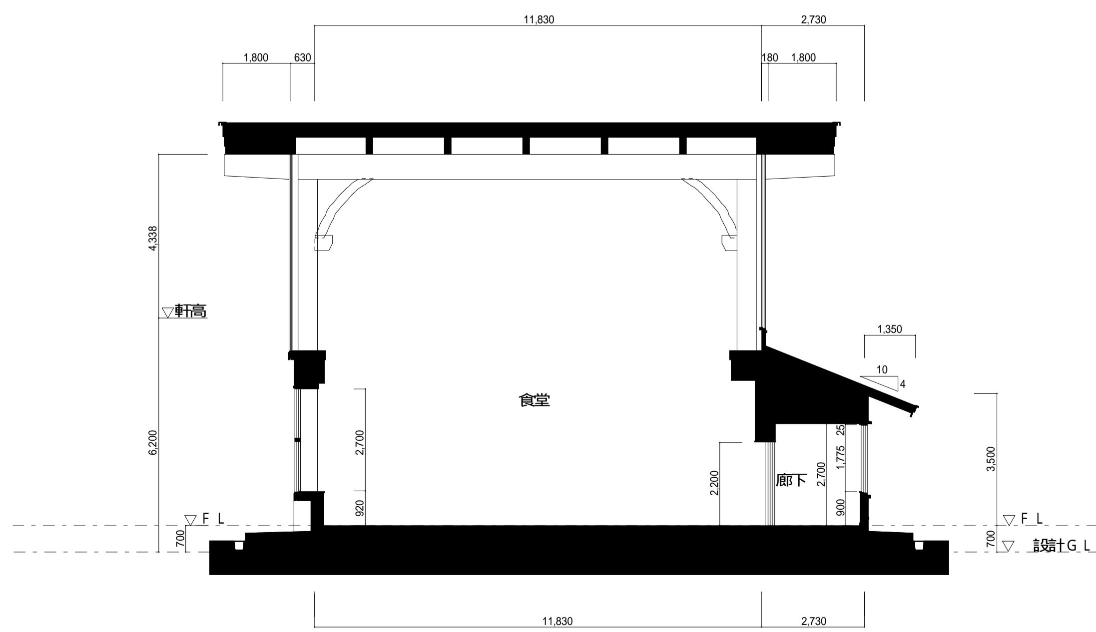
食堂棟 C-C断面図
