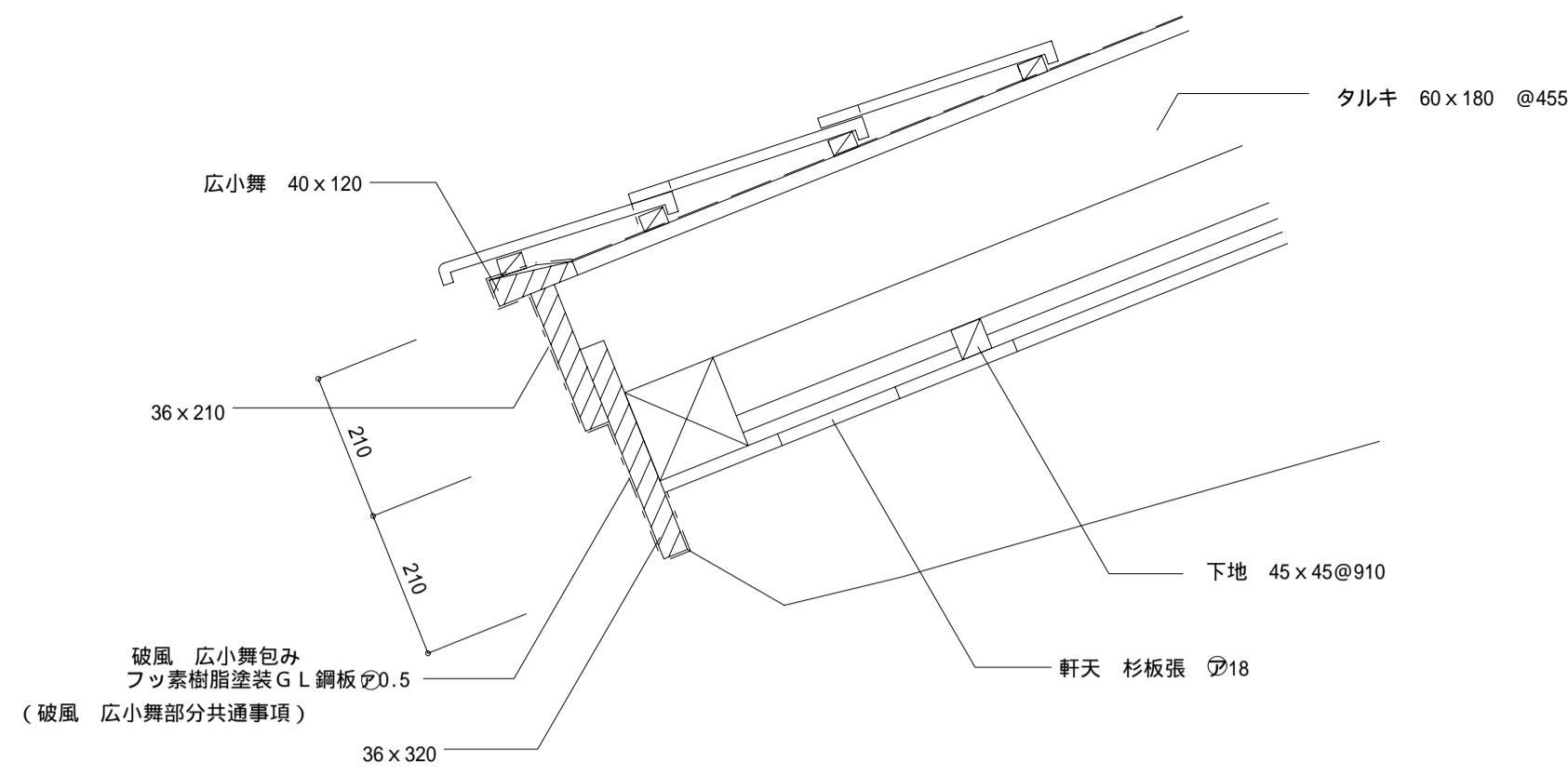
軒先詳細 1:10
