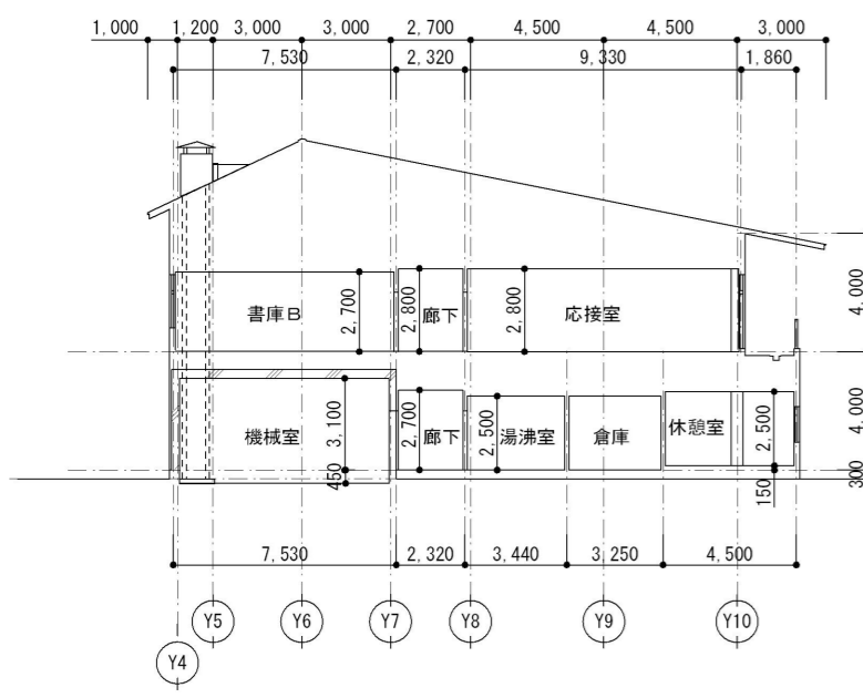
B~B 断面図 S=1:200
