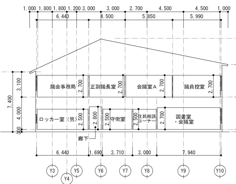
E~E 断面図 S=1:200
