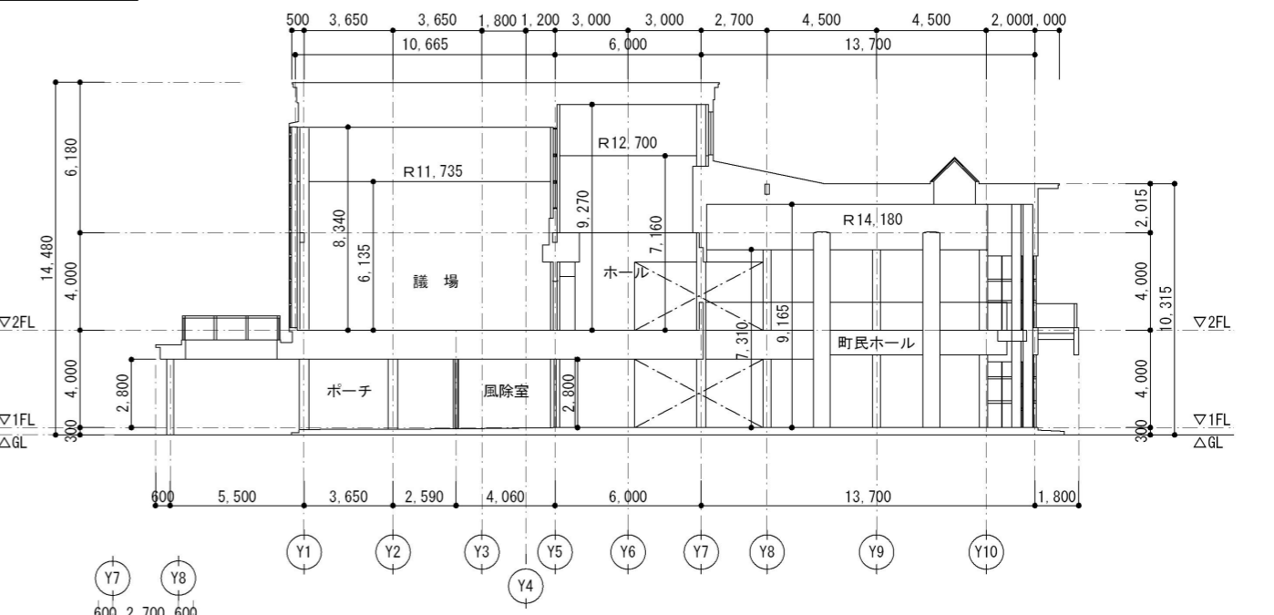
D~D 断面図 S=1:200
