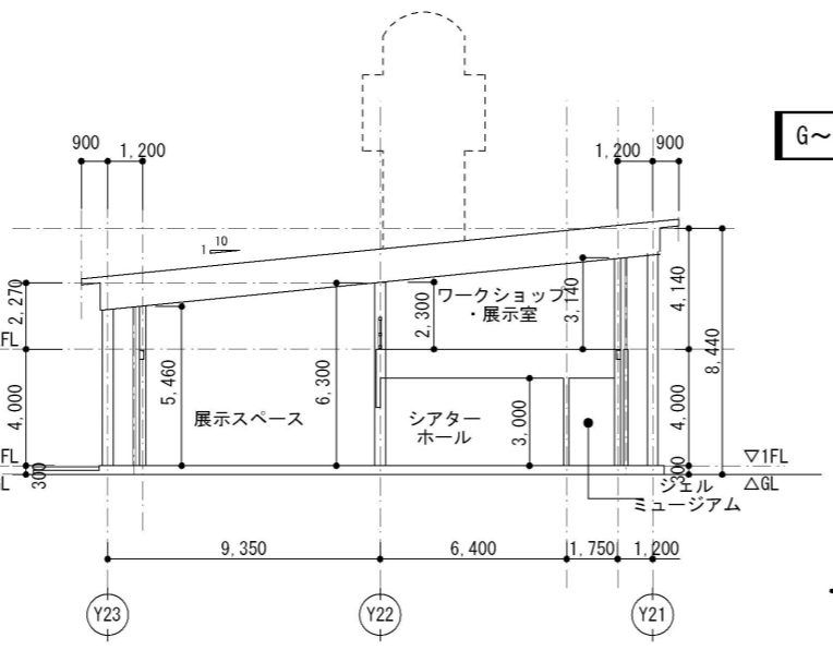
F~F 断面図 S=1:200
