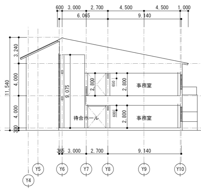
C~C 断面図 S=1:200
