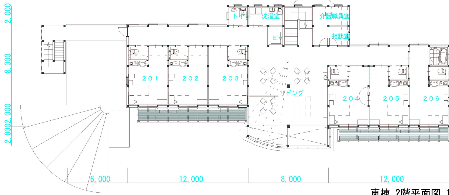
東棟 2階平面図 1 : 300
