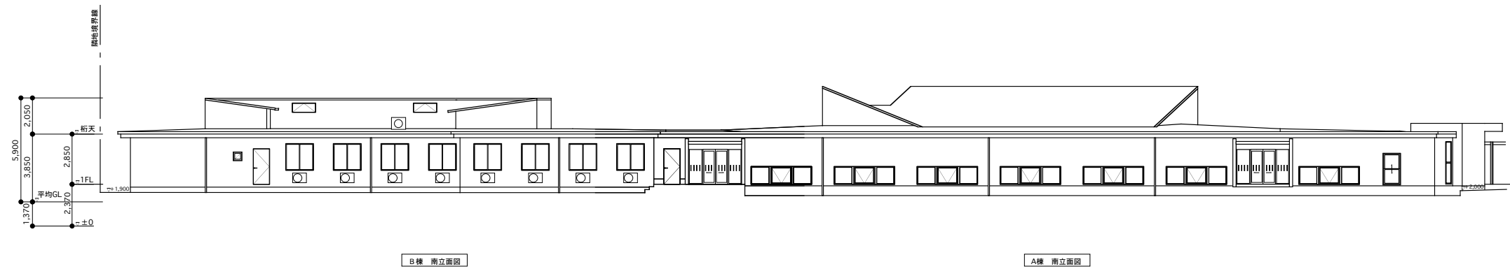
A棟 南立面図
