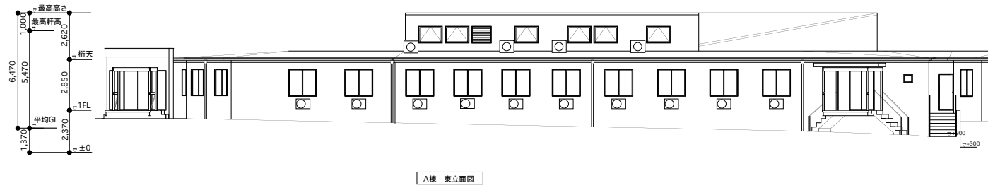
A棟 東立面図
