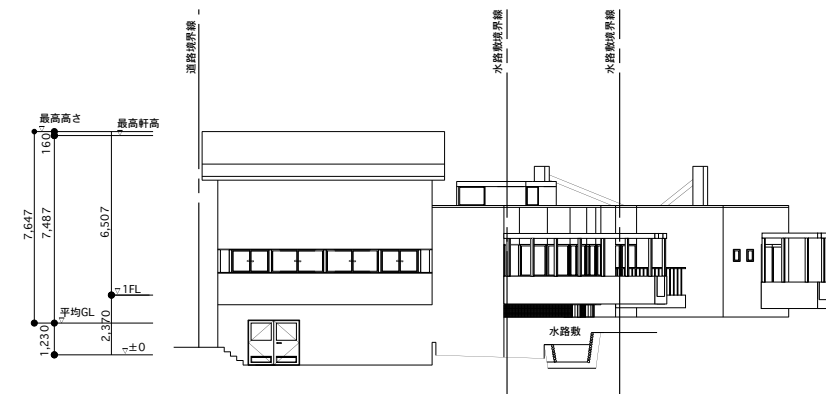
D棟 西立面図
