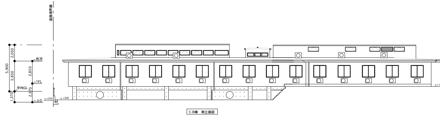
C-B棟 南立面図
