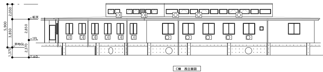
C棟 西立面図
