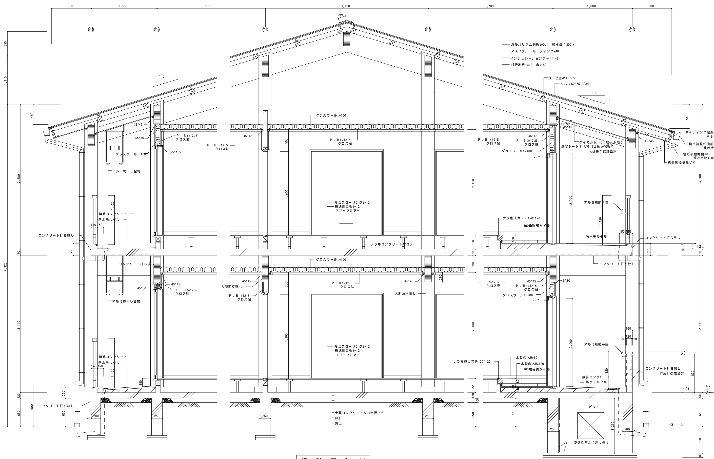
矩計図 S=1:30
