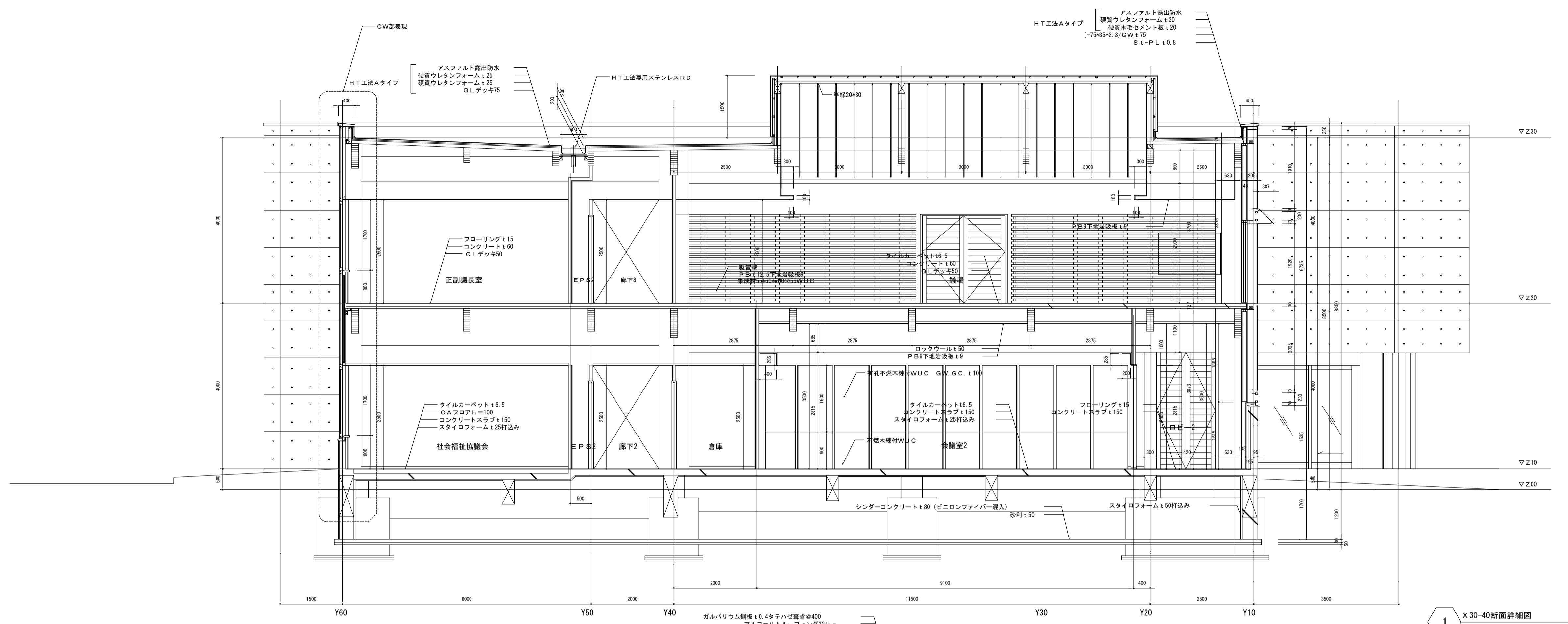
1 X30-40断面詳細図 縮尺 1:60
