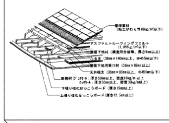
屋根の30分耐火構造 (認定番号FP030RF-0054)
