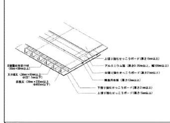
床の1時間耐火構造 (認定番号FP060FL-0016)
