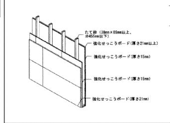
間仕切壁耐力壁の1時間耐火構造 (認定番号FP060BP-0006)
