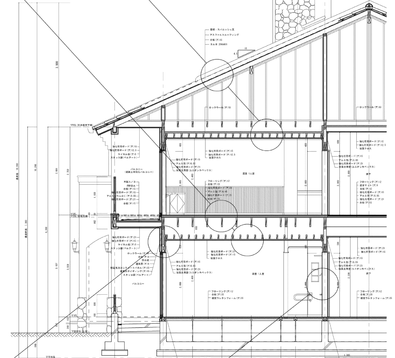
外壁耐力壁の1時間耐火構造 (認定番号FP060BE-0006)
