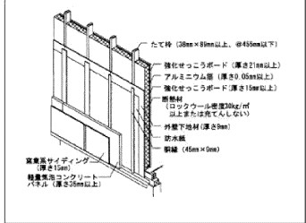
外壁耐力壁の1時間耐火構造 (認定番号FP060BE-0006)
