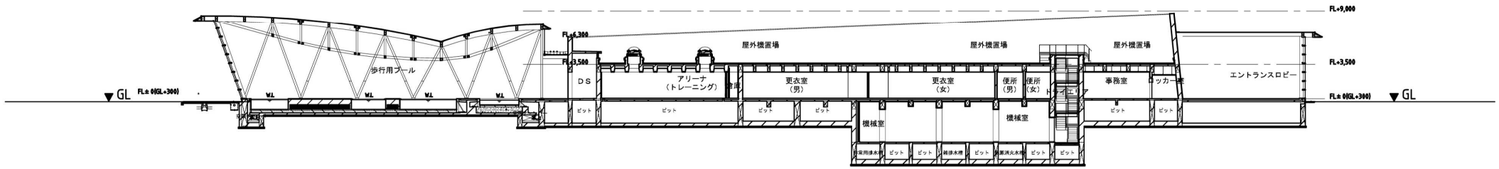
断面図-1 (歩行用プール及び事務室関係)
