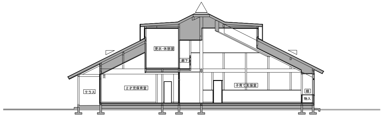
南北断面図 S.1:100
