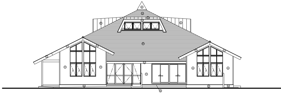
東立面图 S.1:100
