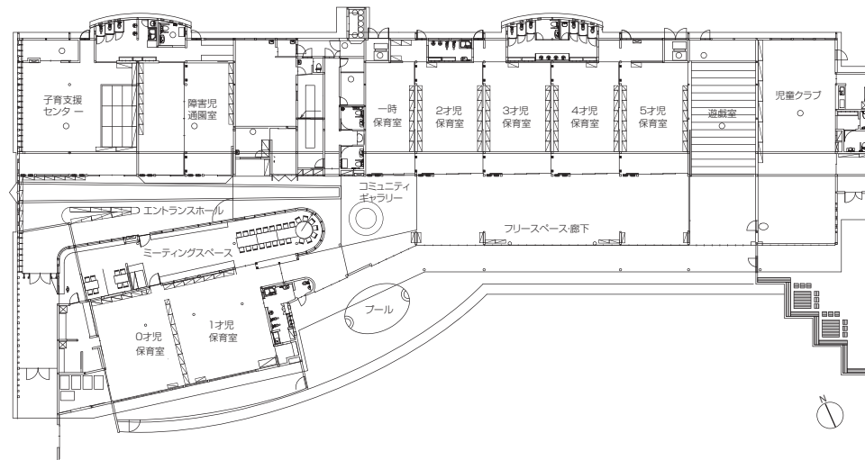
1階平面 縮尺 1/600
