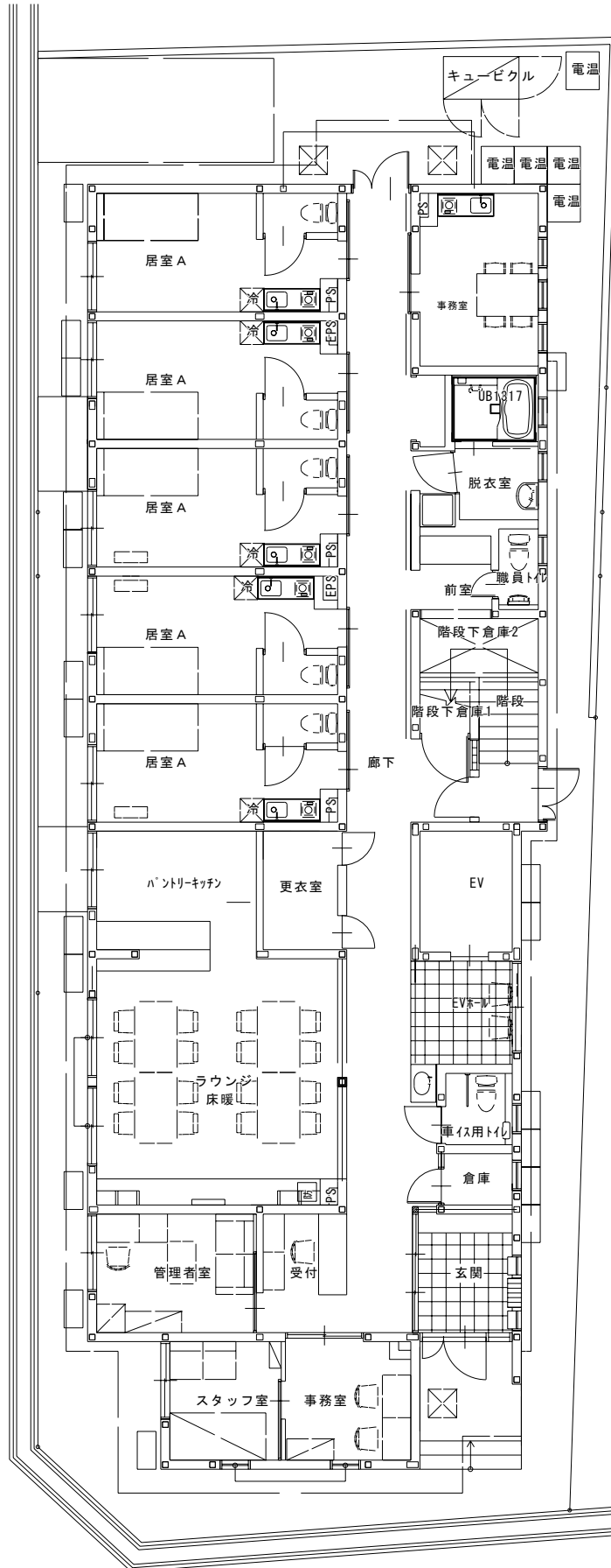
配置図兼1階平面図 S:1/100
