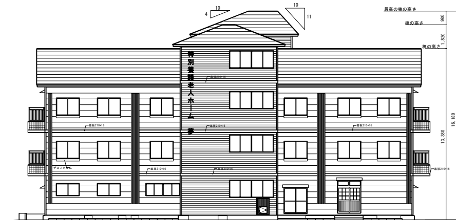
南側立面図 1:150
