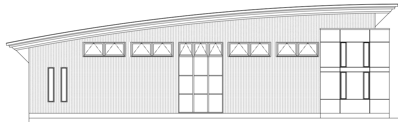
南側立面図
