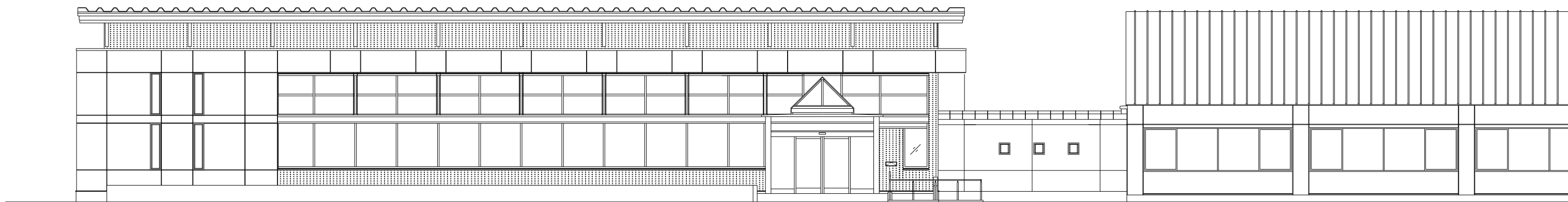
東側立面図
