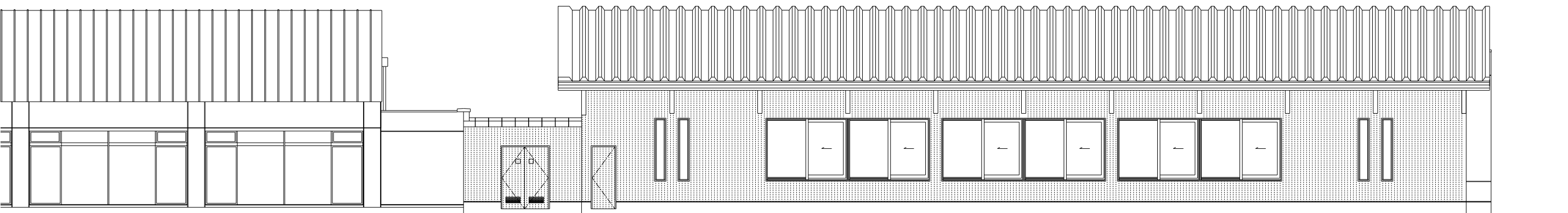
西側立面図
