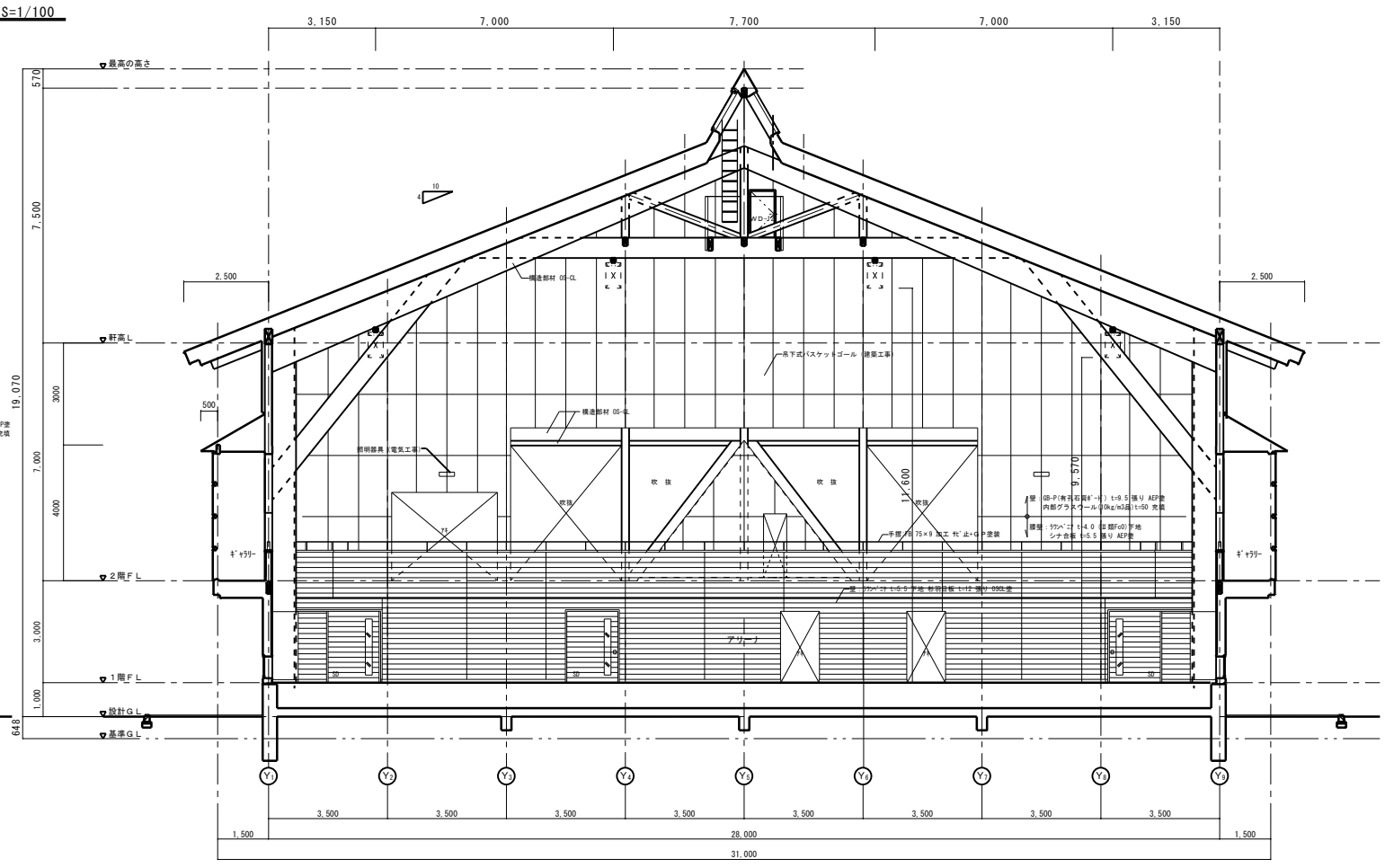
C~C' 断面図 S=1/100
