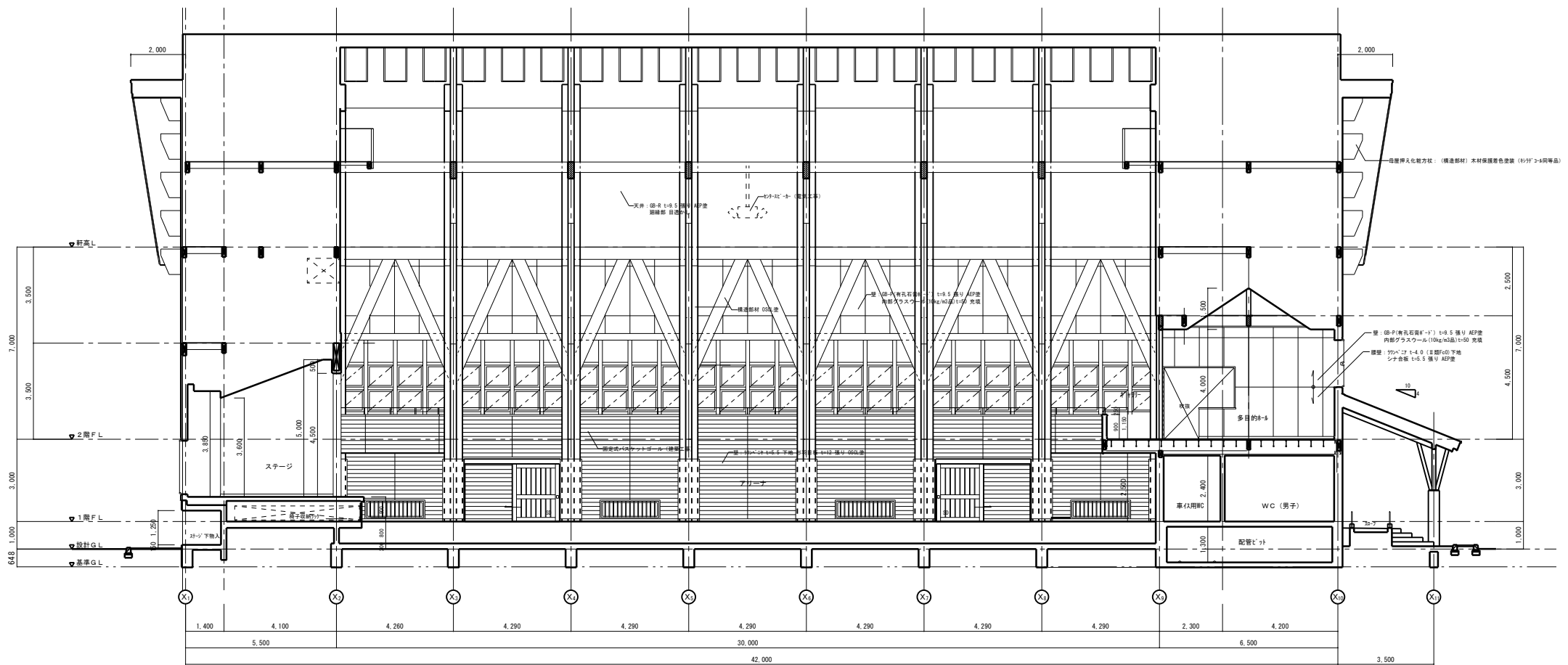
A~A' 断面図 S=1/100
