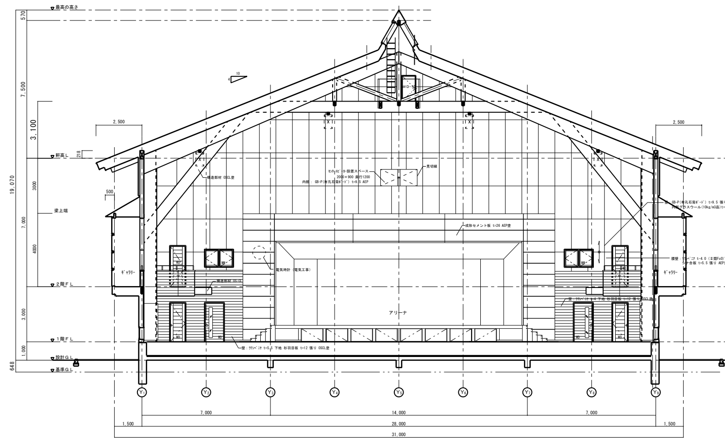
B~B' 断面図 S=1/100
