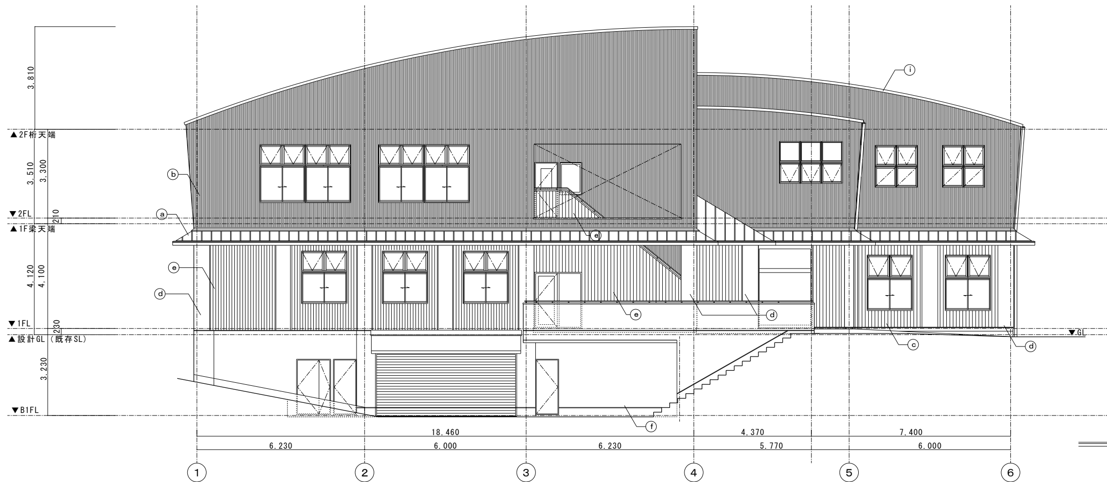
南側立面図
