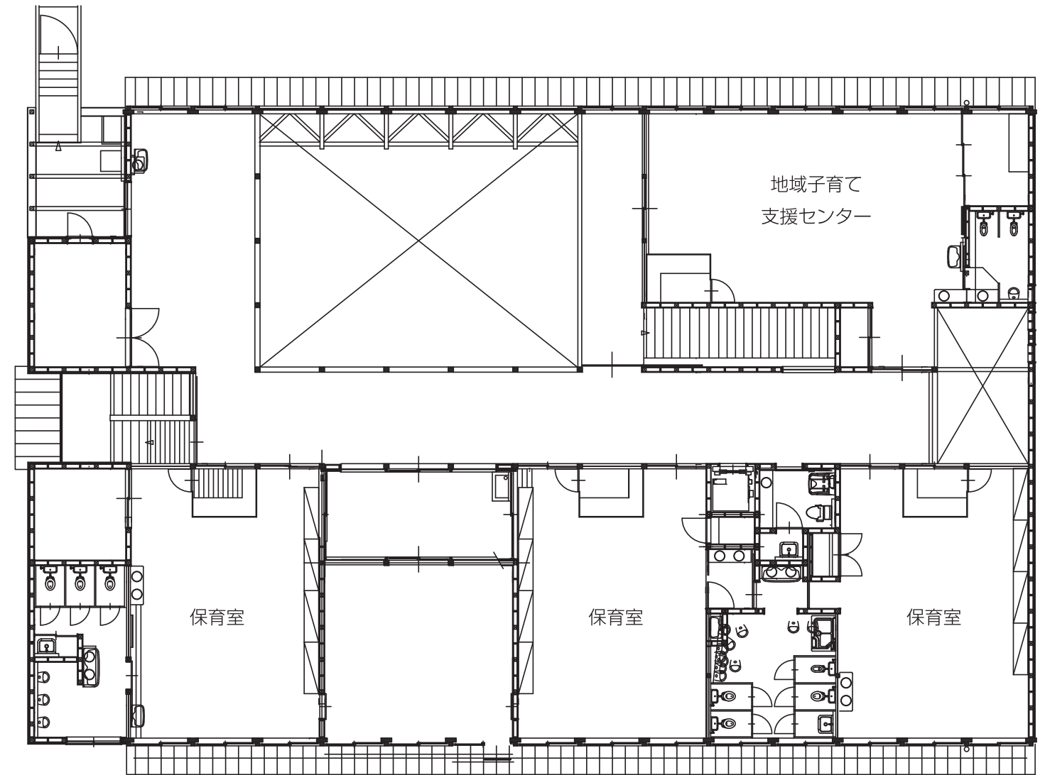
2階平面
