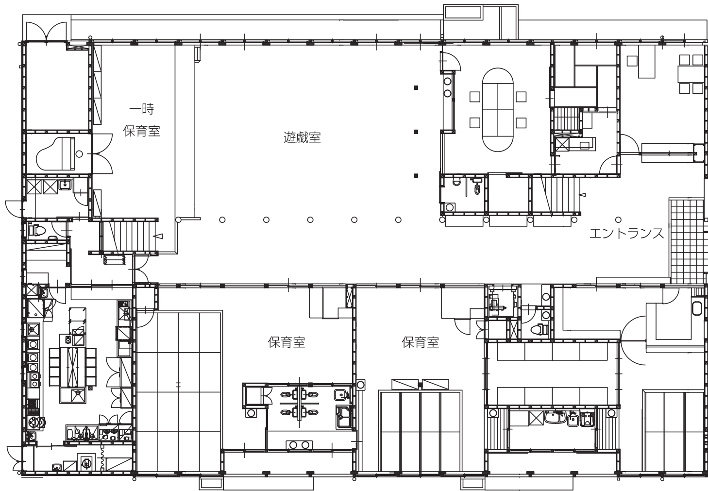
1階平面
