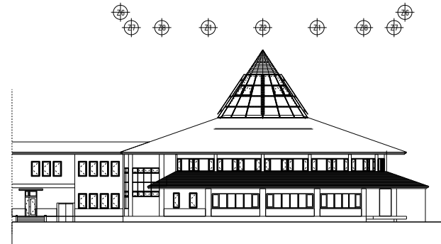
教務棟立面図
