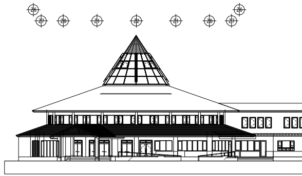
教務棟立面図
