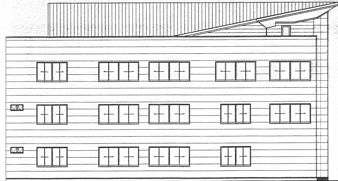
東側立面図
