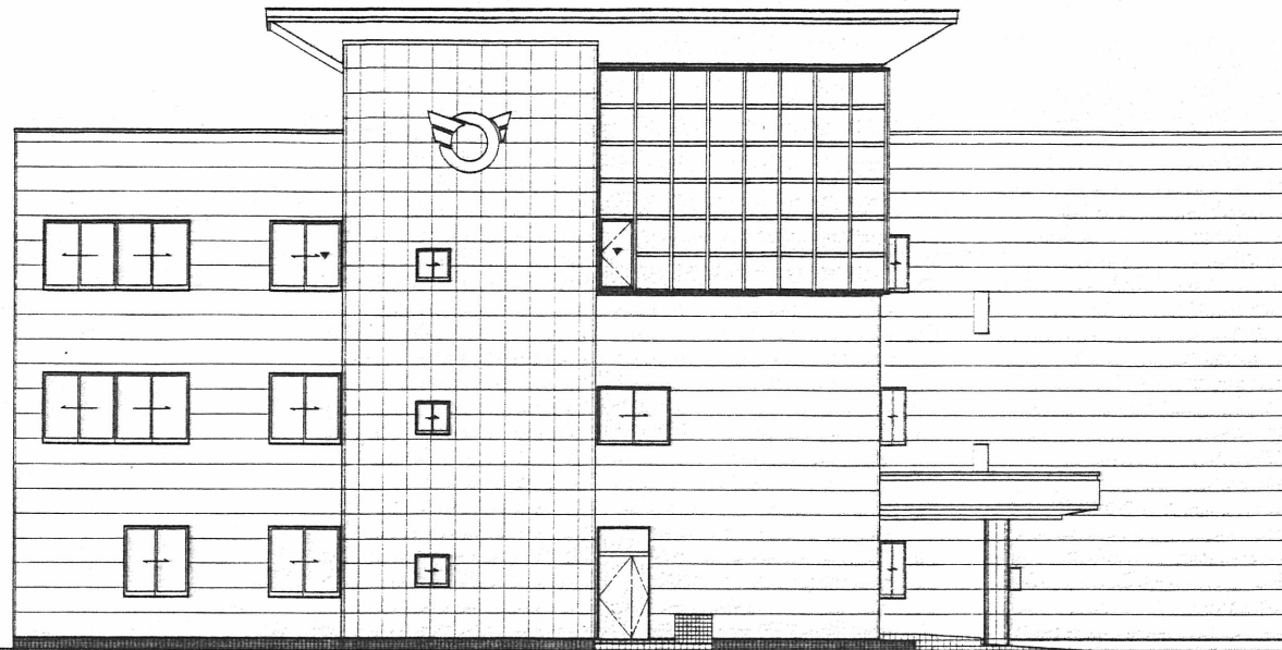
北側立面図
