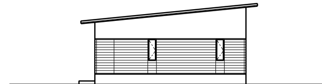
B面 立面图
