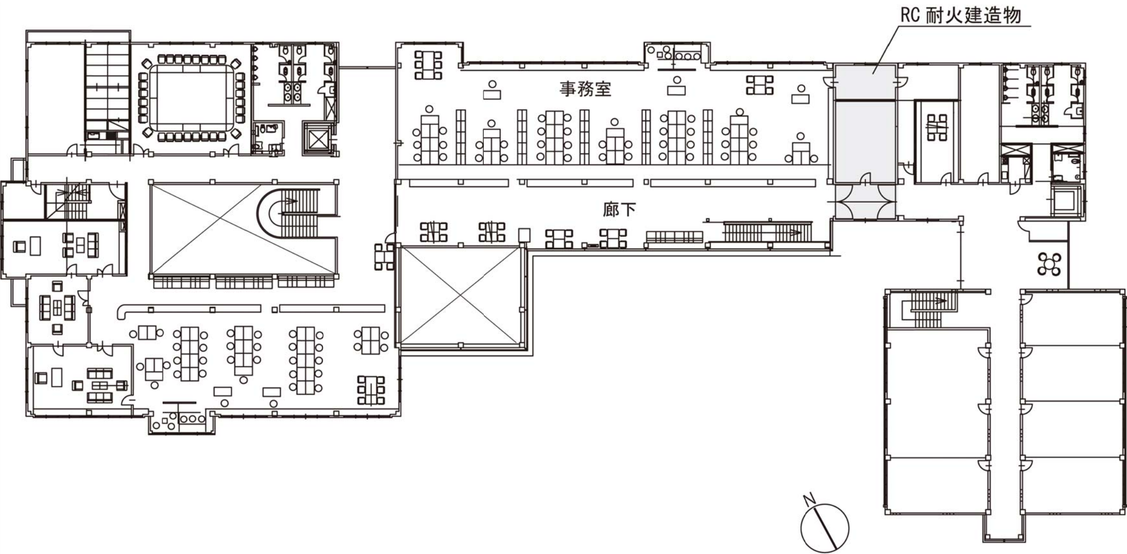
2階平面
