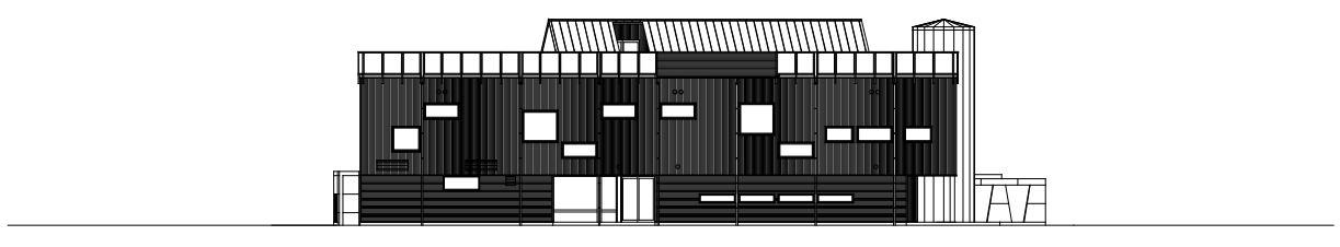
西立面圖
