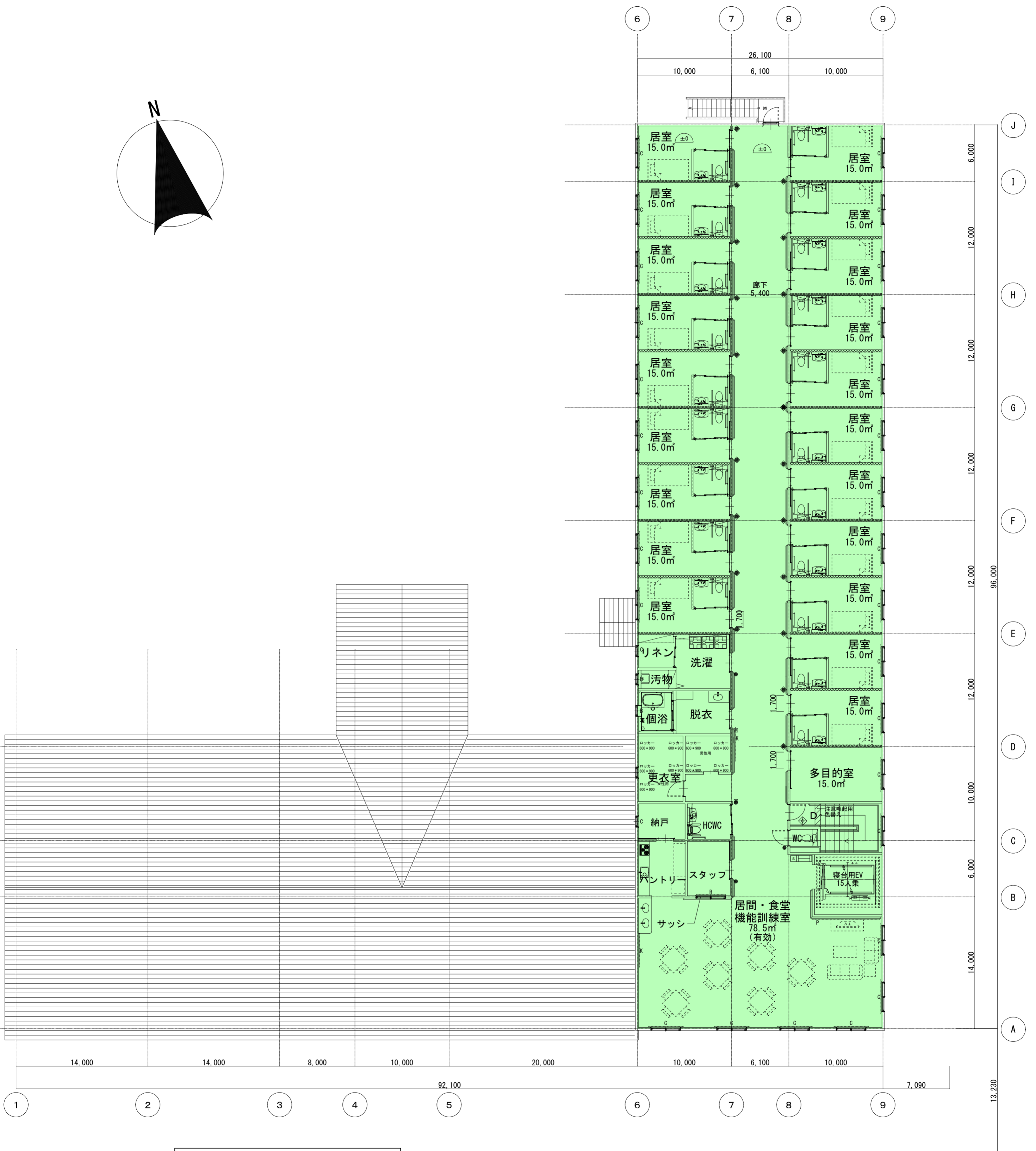
2階平面図 1/200 ×100% (A2) ×71% (A3)
