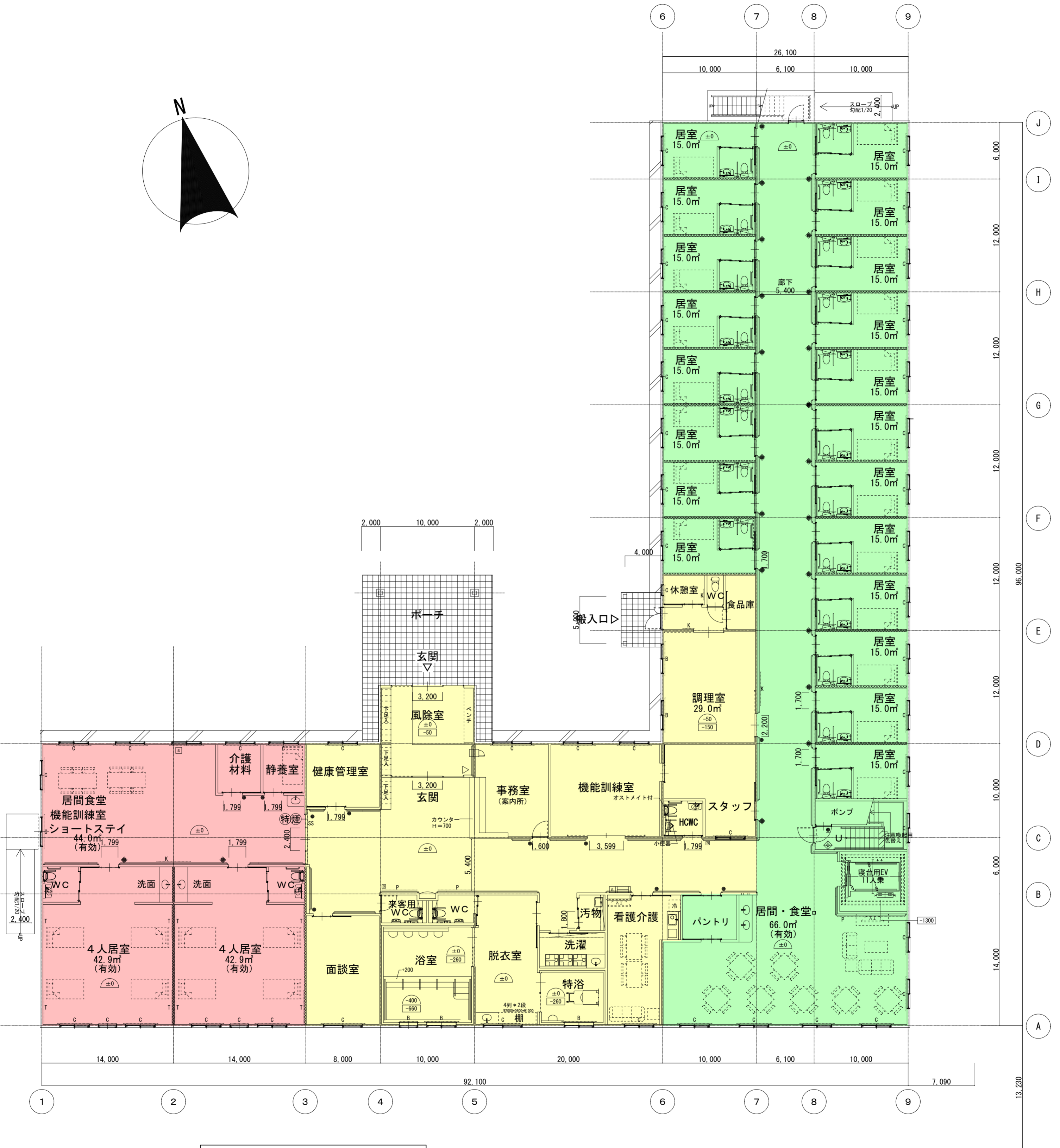
1階平面図 1/200 ×100% (A2) ×71% (A3)
