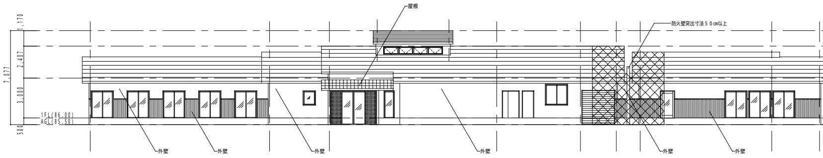
管理棟 南立面図
