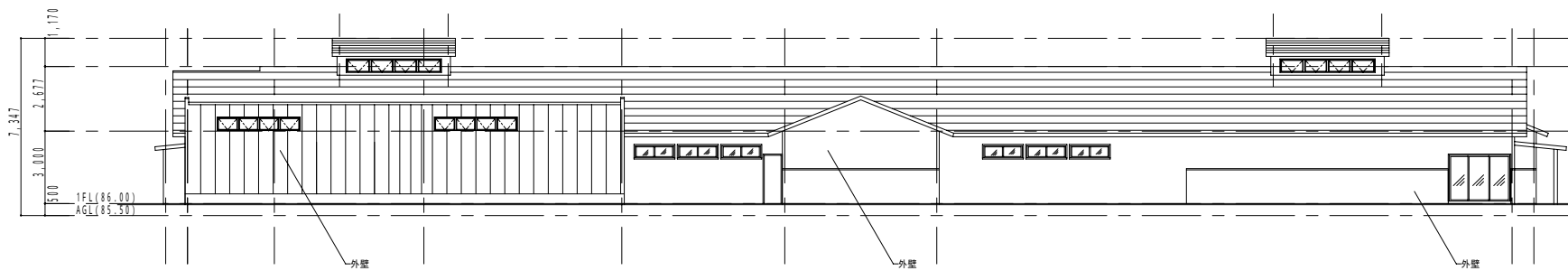
温浴棟 北立面图
