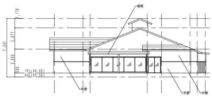
温浴棟 西立面图
