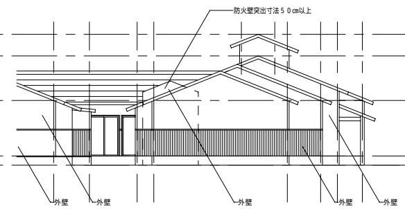
管理棟 西立面図
