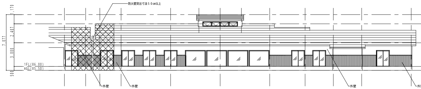
管理棟 北立面図
