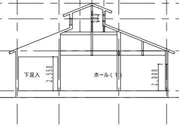
管理棟 断面図
