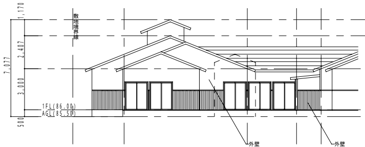
管理棟 東立面図
