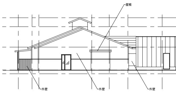
温浴棟 東立面图
