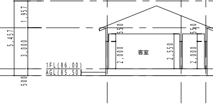
管理棟 断面図
