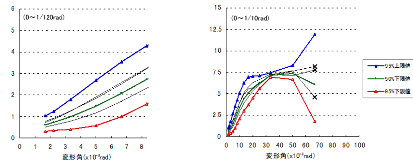
H-4-②の荷重-変形角包絡線
