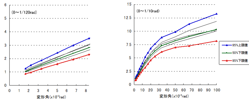
H-4-③の荷重-変形角包絡線
