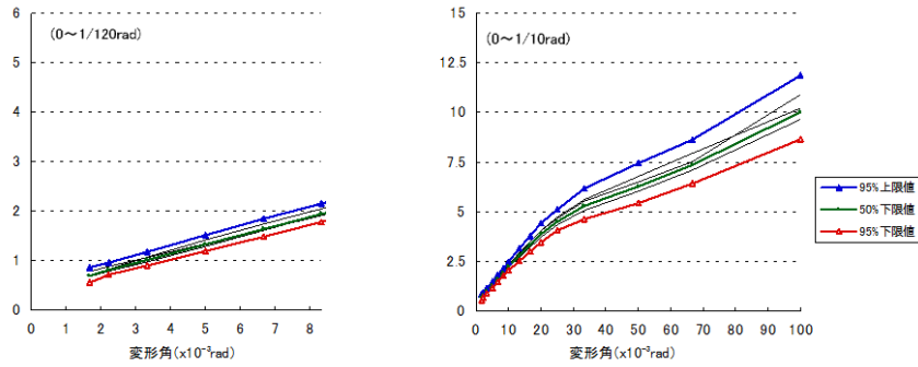
H-4-①の荷重-変形角包絡線
