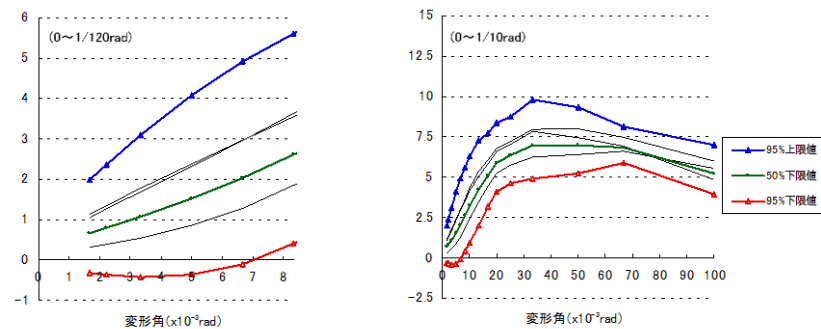
H-4-④の荷重-変形角包絡線
