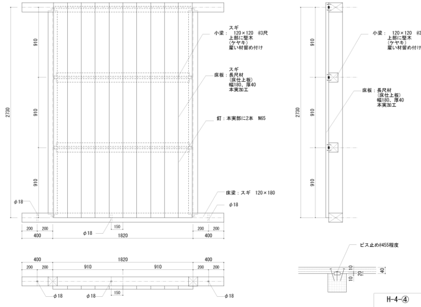
H-4-④の試験体図 (mm)
