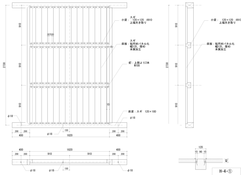
H-4-①の試験体図 (mm)
